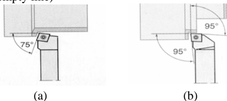
Fig. 1. Tool holder used: (a) PCBNR (b) PCLNR.
